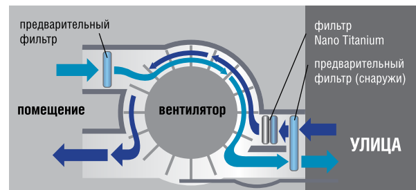
Принцип воздухообмена
